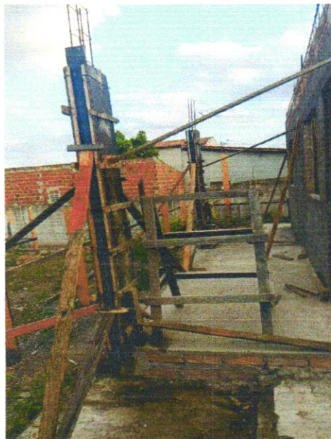
MONTAGEM E CONCRETAGEM DE PILARES
