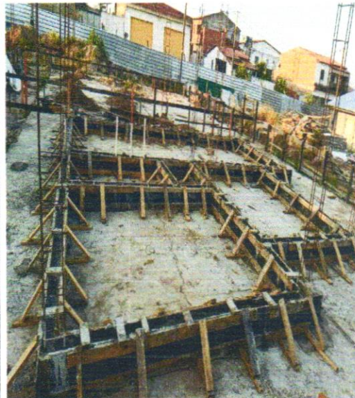
MONTAGEM E CONCRETAGEM DE BALDRME
