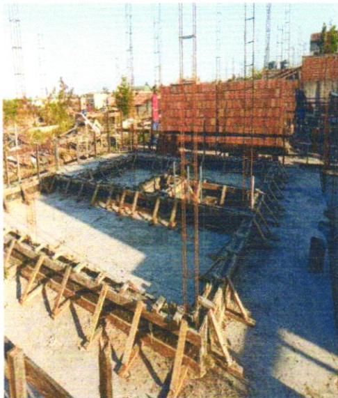
ARMAÇÃO DE SAPATA, VIGA BALDRAME E PILAR
